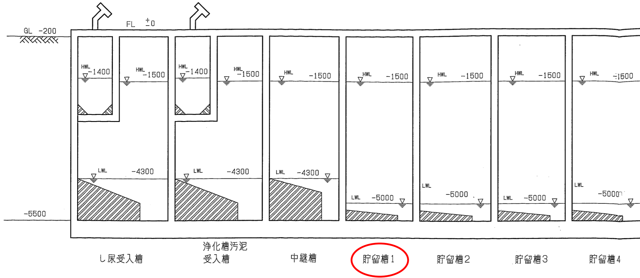
水位高低図
